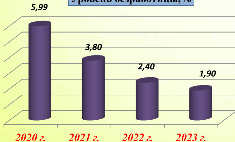
Уровень безработицы, %
